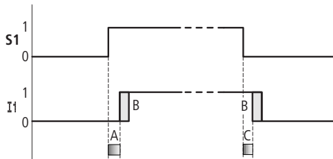
Abbildung 84: Schaltverhalten bei abgeschalteter Eingangsverzögerung
