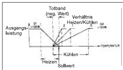
Bild 7.12: Heizen/Kühlen-Funktion (db&lt;0)
