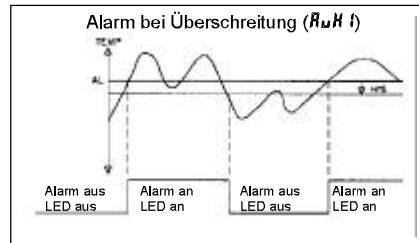
Bild 7.2: Alarm bei Überschreitung
