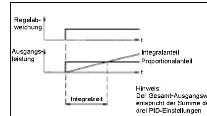
Bild 8.2: Integralzeit
