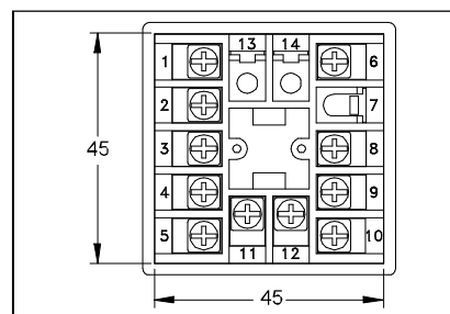
Bild 3.4: Geräterückseite (Angaben in mm)
