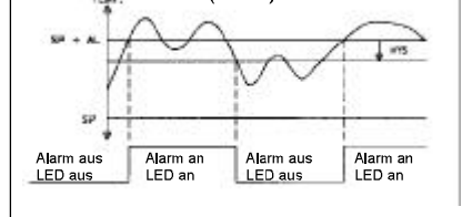
Bild 7.4: Alarm bei Abweichung über (AL pos.)
