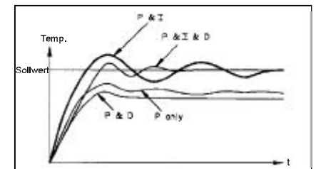
Bild 8.4: Typische Sprungantworten
