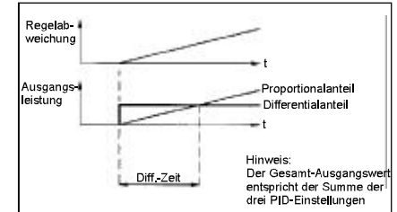
Bild 8.3: Differentialzeit
