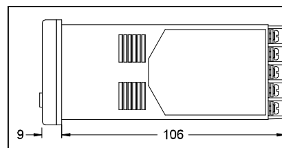
Bild 3.3: Seitenansicht (Angaben in mm)
