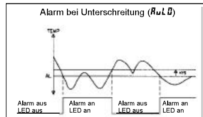
Bild 7.3: Alarm bei Unterschreitung
