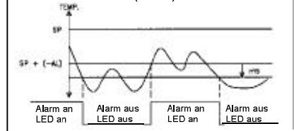
Bild 7.5: Alarm bei Abweichung unter (AL neg.)
