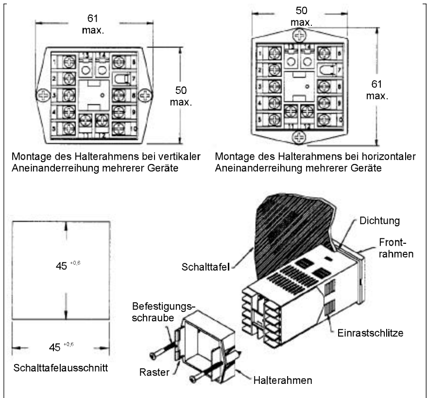
Bild 4.1: Schaltfelaufbau (Angaben in mm)
