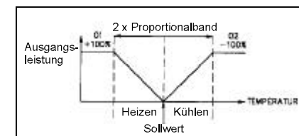
Bild 7.10: Heizen/Kühlen-Funktion (db=0)
