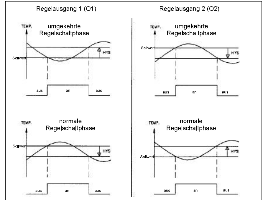
Bild 9.2: 2-Punkt-Regelung
