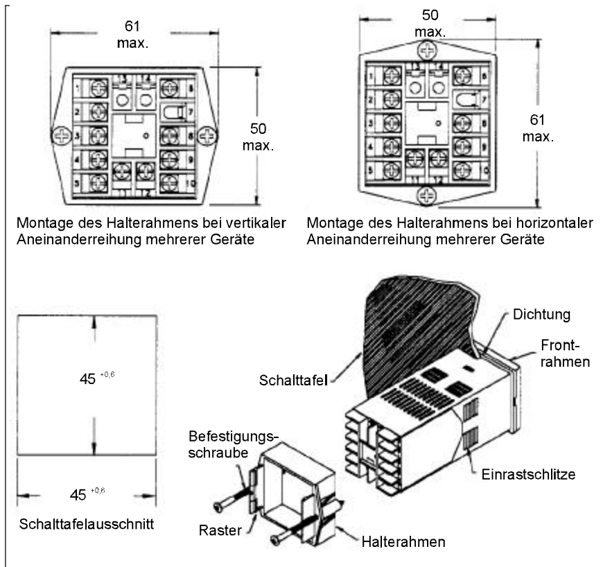
Bild 4.1: Schaltungstafeleinbau (Angaben in mm)
