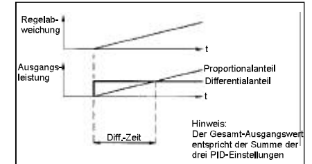
Bild 8.3: Differentialzeit
