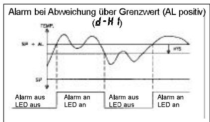
Bild 7.4: Alarm bei Abweichung über (AL pos.)
