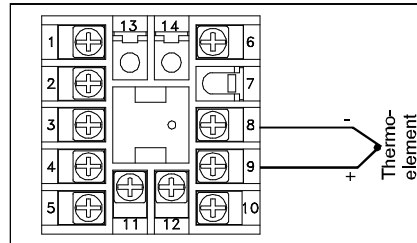
Bild 5.1: Anschluß eines Thermoelementes
