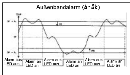
Bild 7.7: Außenbandalarm
